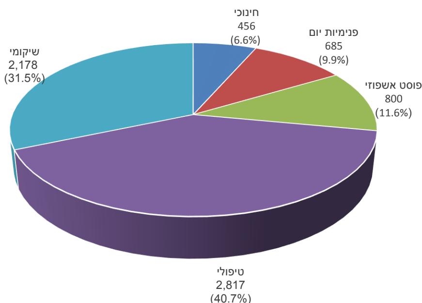
תרשים 1: חניכים לפי תעריף (N = 6,917)
