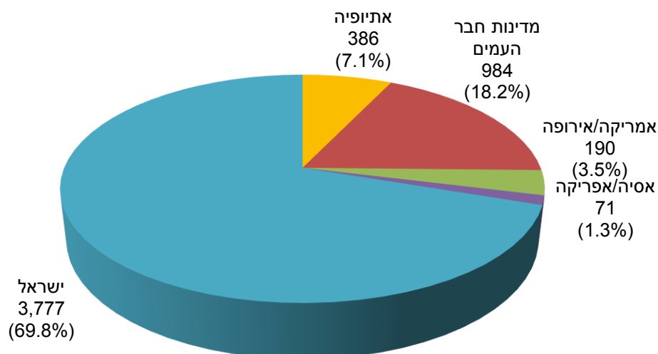
תרשים 9: חניכים לפי ארץ מוצא (N = 5,408)*
